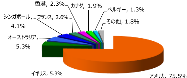
国別構成比率（2020年3月末現在）
