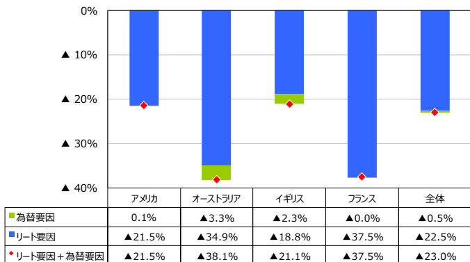
2020年3月の国別収益要因分解
